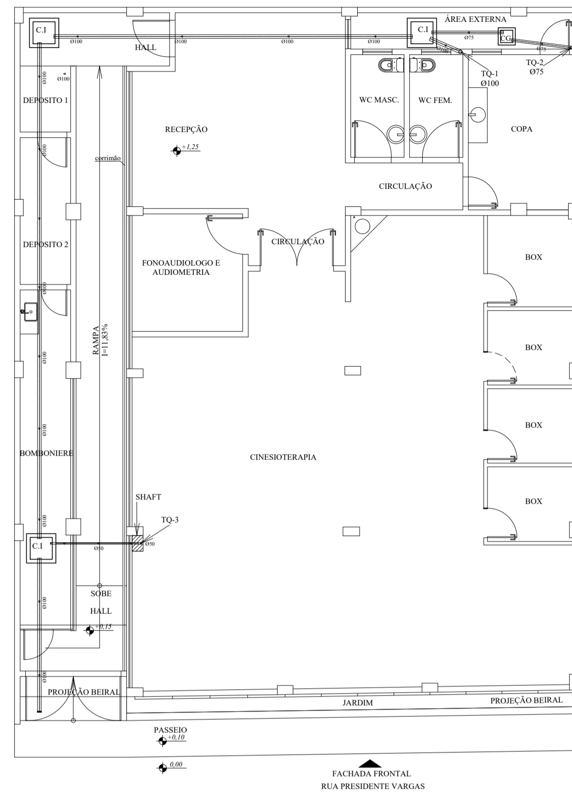
11 PLANTA BAIXA ESGOTO - PAVIMENTO TÉRREO ESCALA : 1/100
