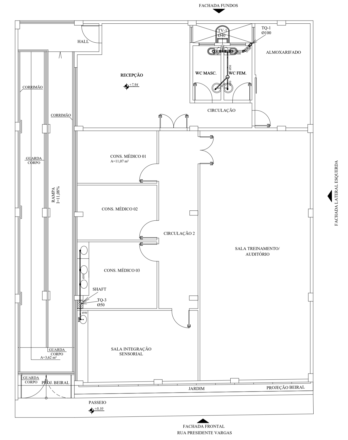
13 PLANTA BAIXA ESGOTO - 2º PAVIMENTO ESCALA : 1/100
