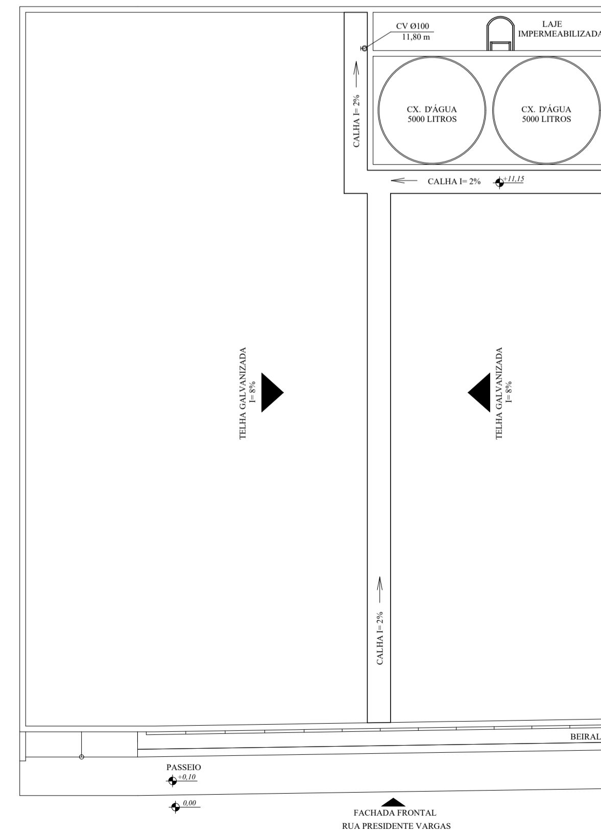
15 PLANTA BAIXA PLUVIAL - COBERTURA ESCALA : 1/100
