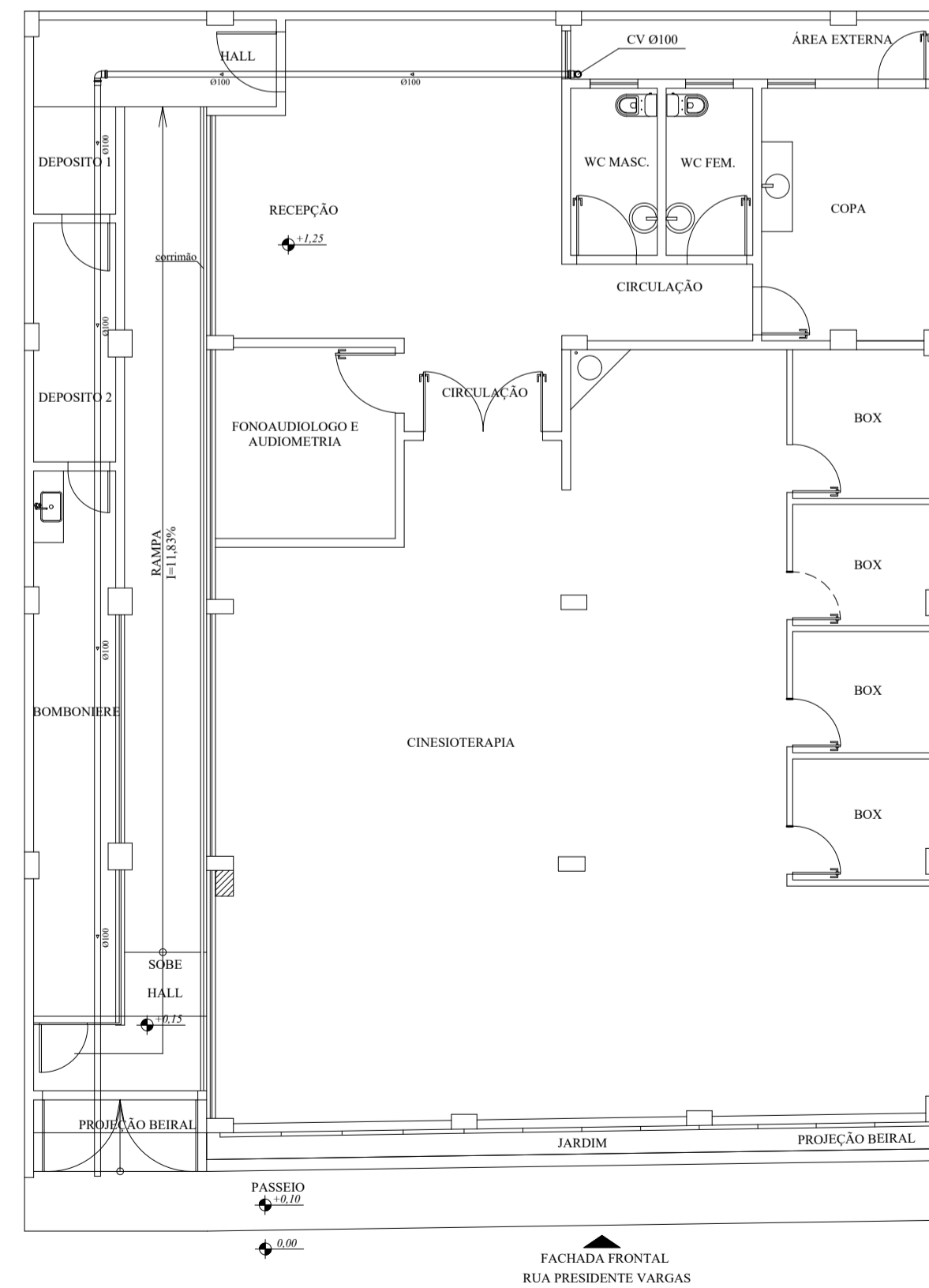
14 PLANTA BAIXA PLUVIAL - TÉRREO ESCALA : 1/100
