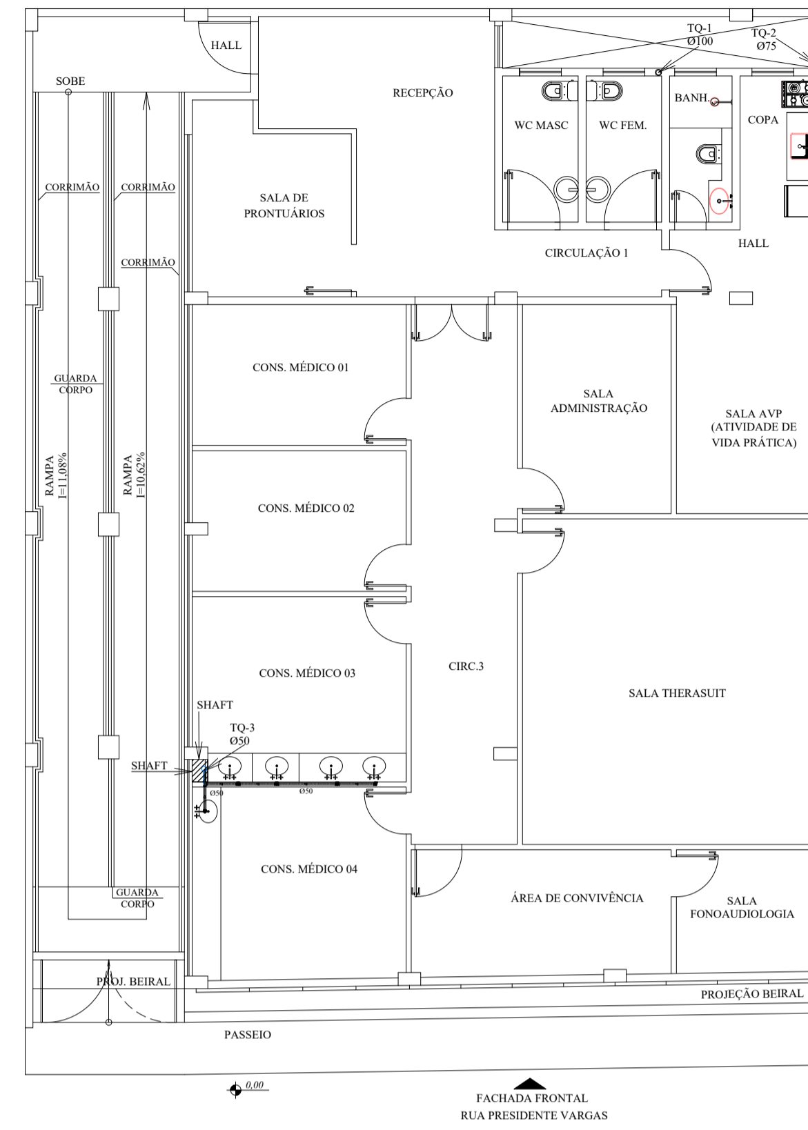
12 PLANTA BAIXA ESGOTO - 1º PAVIMENTO ESCALA : 1/100
